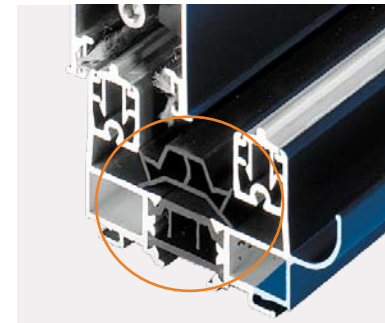
Le bouclier thermique permet de renforcer l'isolation de la baie
